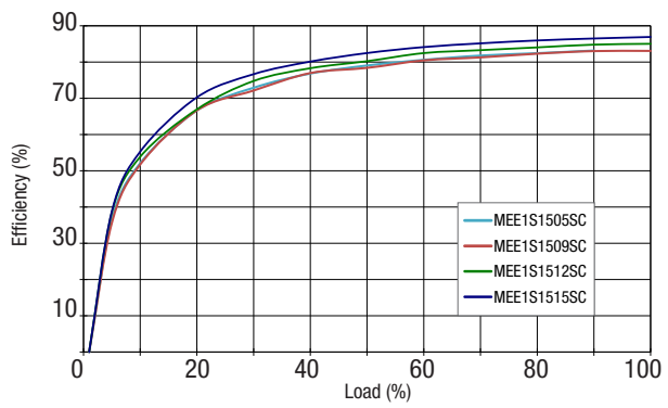
15V Input
