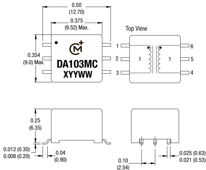
6 Pin SM
