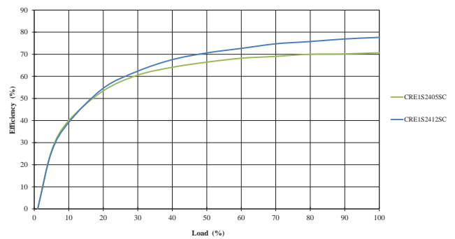
24V Inputs
