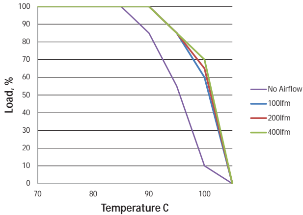
MTC2S1203MC - 18Vin
