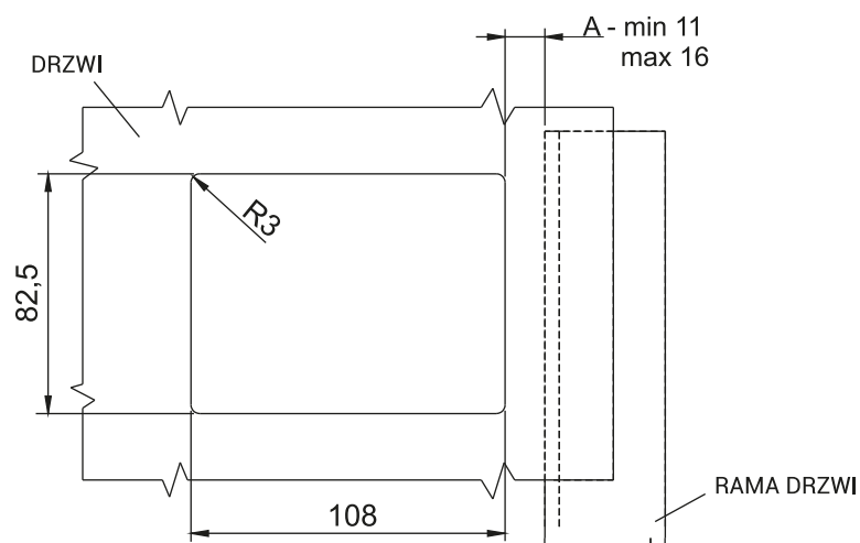
Otwór montażowy
