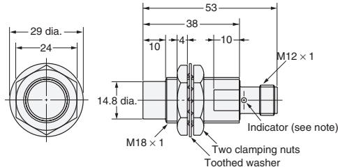
Fig. 24 : E2E-X14MD□-M1(G)/E2E-X10ME□-M1/F□-M1 E2E-X10MY□-M1
