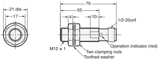
E2E2-X2Y□-M4
