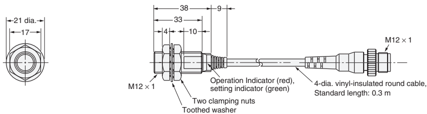
Fig. 29 : E2E-X3D1-M1GJ E2E-X3D1-M1J-T
