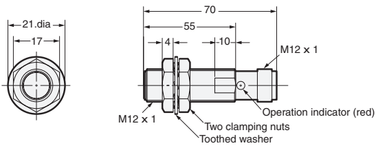
E2E2-X2Y□-M4
