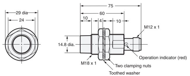
E2E2-X10MY□-M4
