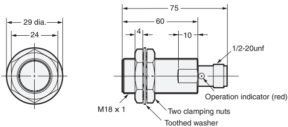
E2E2-X5Y□-M4
