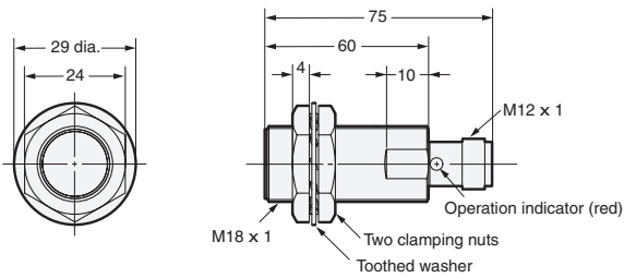
E2E2-X5C□-M1/B□-M1
