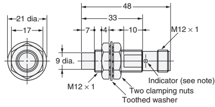
Fig. 20 : E2E-X8MD□-M1(G) E2E-X5ME□-M1/F□-M1
