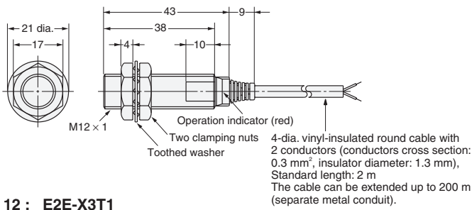
Fig. 12 : E2E-X3T1
