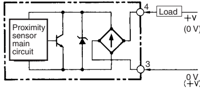
E2E-X□D1-M1J-T No Polarity
