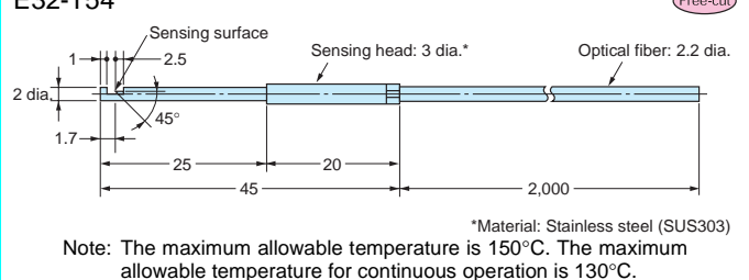
E32-T54
