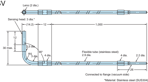
E39-F1V
