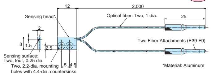
E32-D25XB
