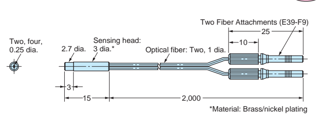
E32-D15XB
