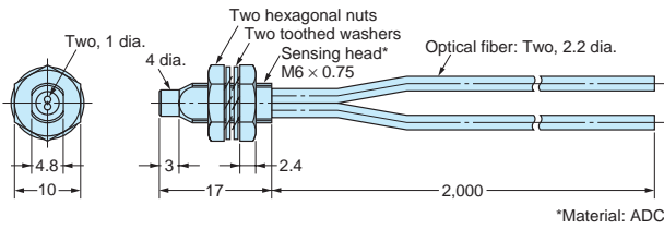
E32-DC200 E32-D11R
