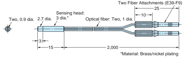
E32-D22L
