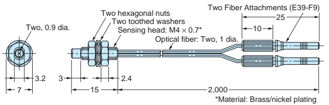
E32-D21L
