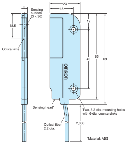
E32-T16J E32-T16JR
