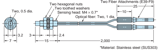
E32-DC200E E32-D21R
