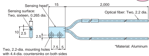
E32-D15XB
