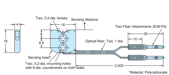
E32-L25A
