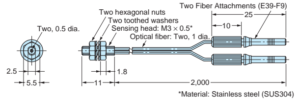
E32-DC200E E32-D21R
