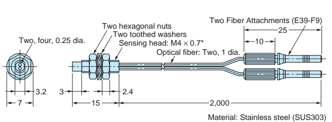
E32-D221B
