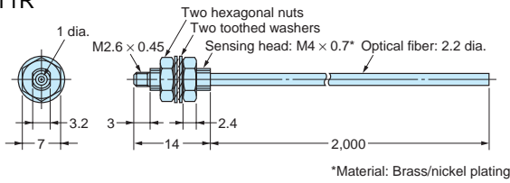
E32-TC200 E32-T11R
