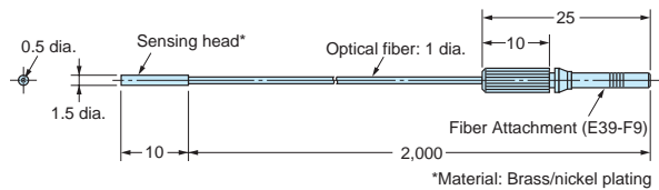
E32-T25X E32-T25XR
