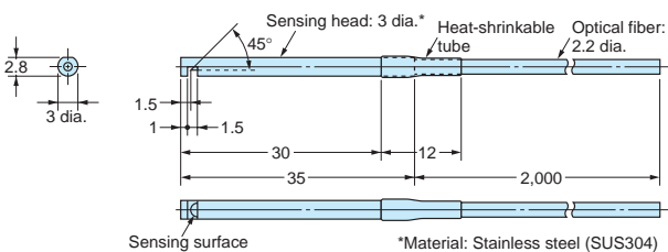
E32-T14L E32-T14LR
