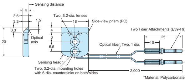
E32-L25
