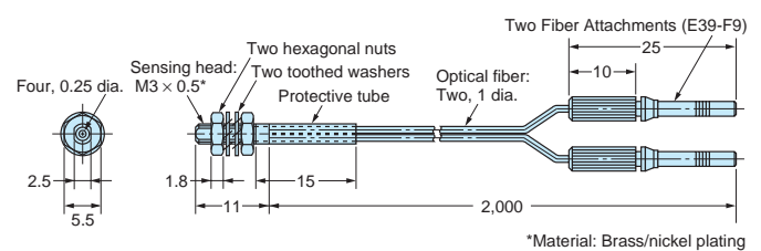
E32-D22B
