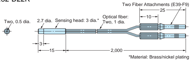
E32-D22 E32-D22R
