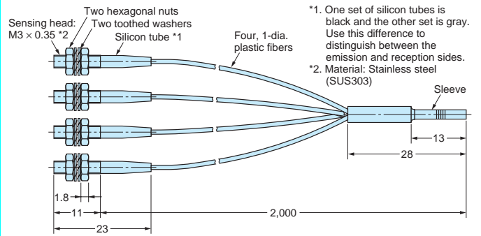
E32-T16
