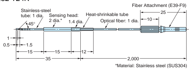
E32-T24 E32-T24R
