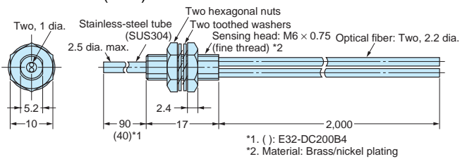
E32-D14L E32-D14LR
