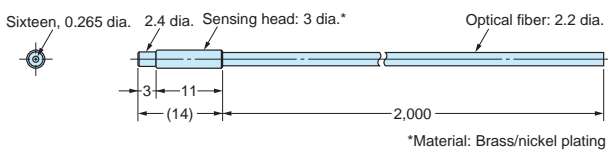
E32-T12B
