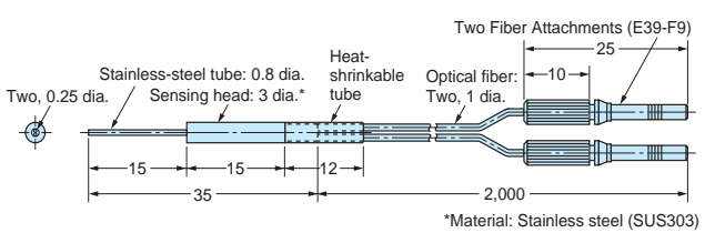
E32-D33
