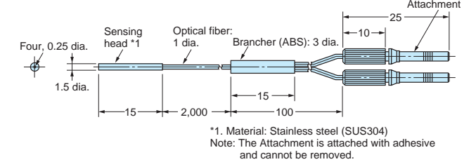
E32-D25XB
