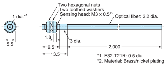
E32-TC200A E32-T21R
