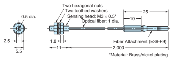
E32-T22 E32-T22R
