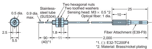
E32-T24 E32-T24R
