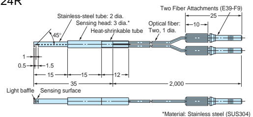
E32-D24 E32-D24R
