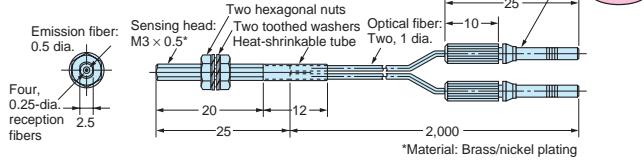
E32-C31
