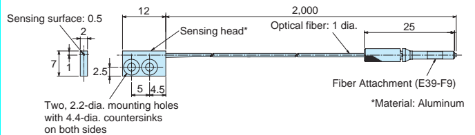
E32-TC200(F4) E32-TC200F(F4R)
