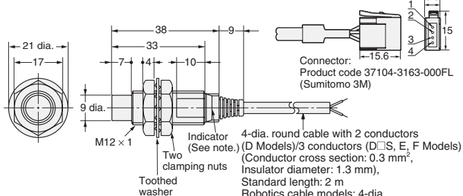
Fig. 9 : E2E-X8MD□ E2E-X5ME□/F□
