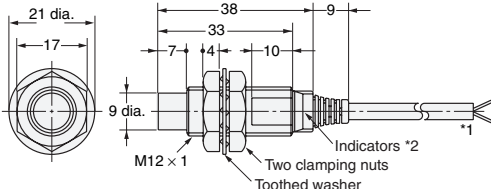
Diagram 10 E2E-X8MD□ E2E-X5ME□/F□
