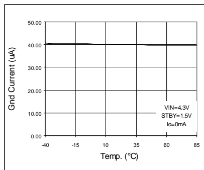
Fig. 160 IIGND vs Temp
