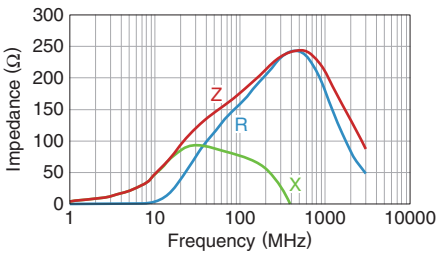
MPZ1608S181ATAH0
