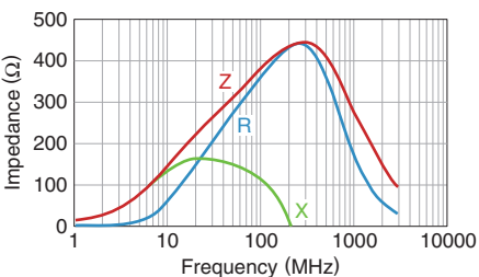
MPZ1608R391ATA00
