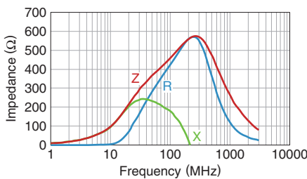
MPZ1608R391ATA00
