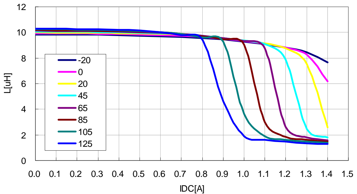
VLF4014ST-100M1R0
