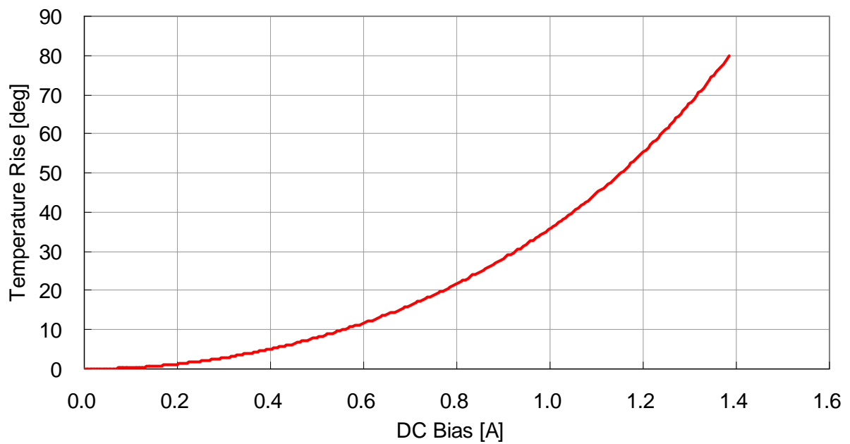
VLF4014ST-100M1R0
