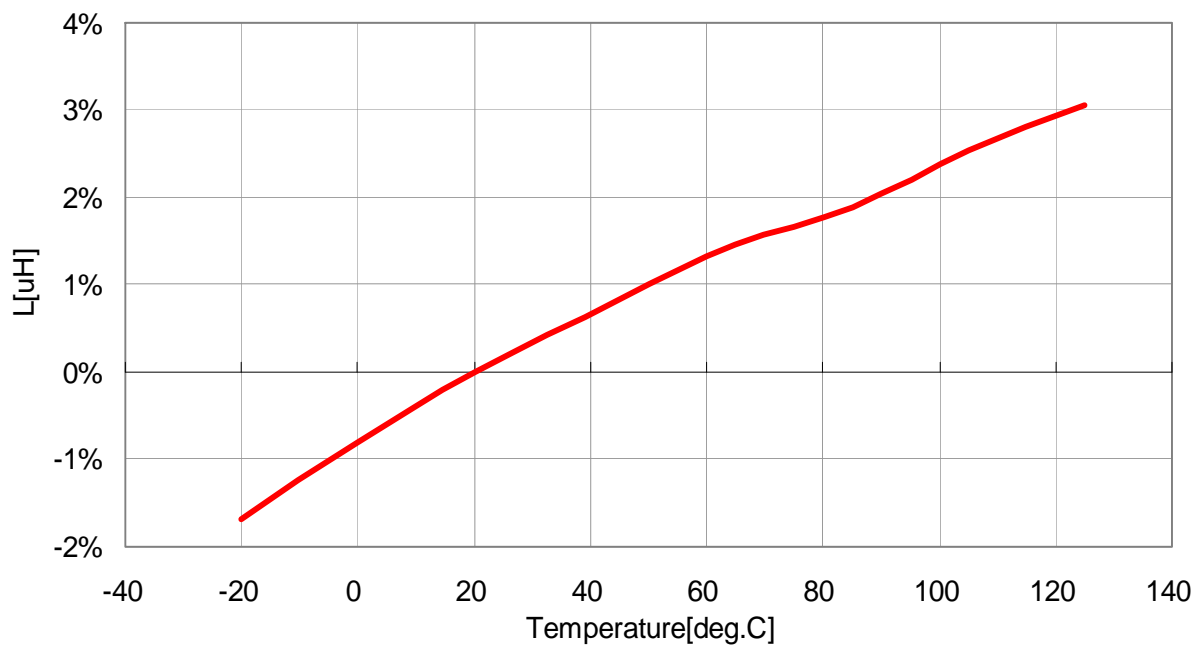
VLF4014ST-100M1R0
