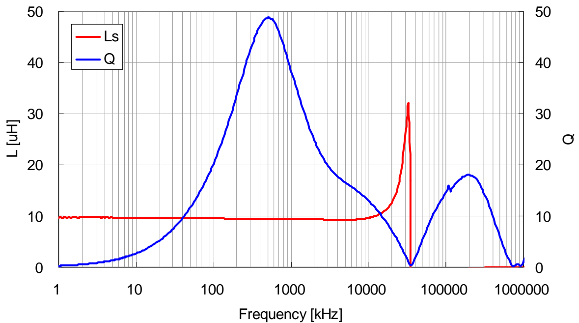
VLF4014ST-100M1R0
