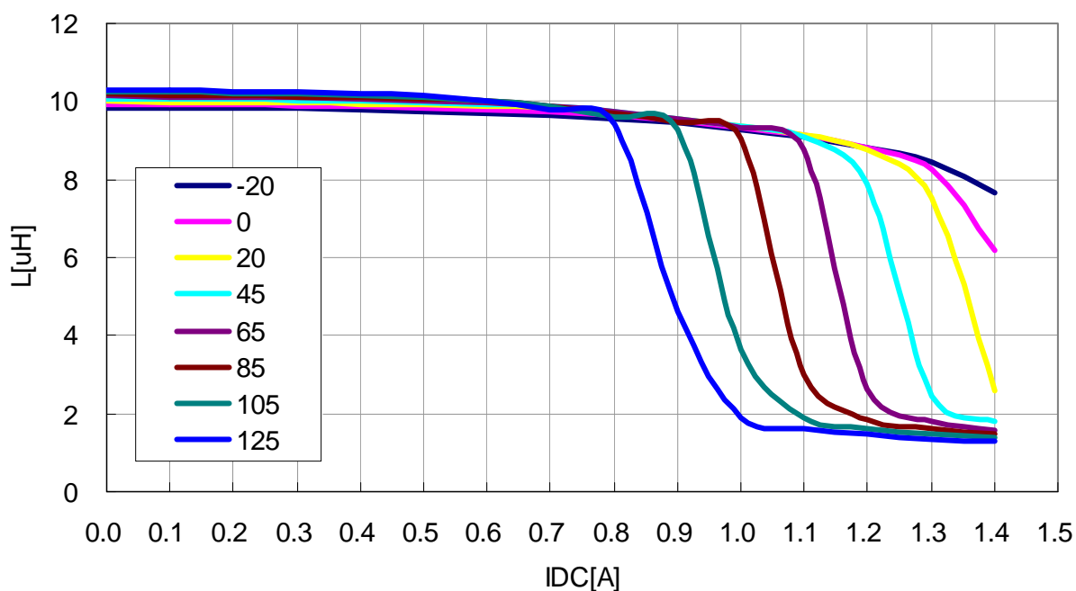
VLF4014ST-100M1R0
