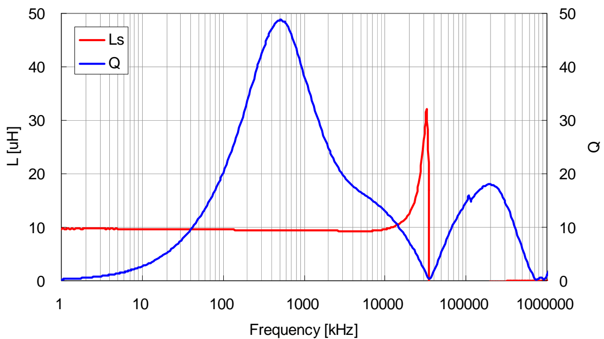
VLF4014ST-100M1R0
