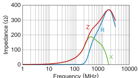
MMZ1608D121CTAH0
