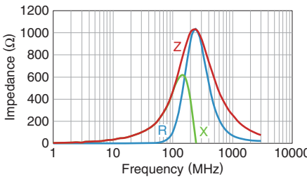
MMZ1608Q471B
