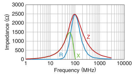
MMZ1608Q331B
