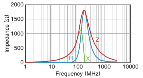
MMZ1608Q102B
