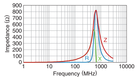
MMZ1608F470BTD25
