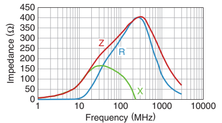
MPZ1608S331ATA00
