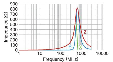
MMZ1608F470BTD25
