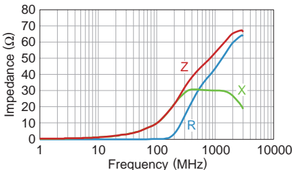
MMZ1608D800CTA00
