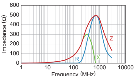
MMZ1608D121BTA00
