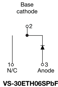
TO-263AB (D²PAK)
