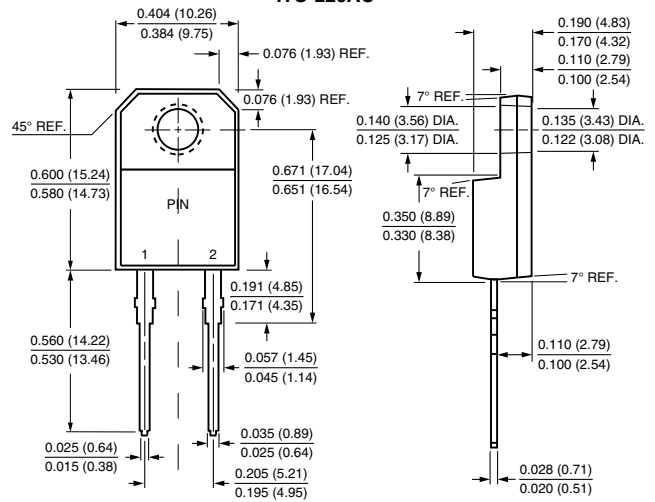
ITO-220AC
