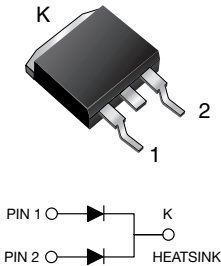
D 2 PAK (TO-263AB)
