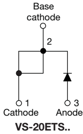
TO-220AC
