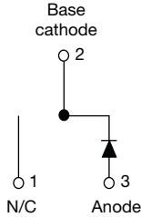
VS-8ETU04SPbF
