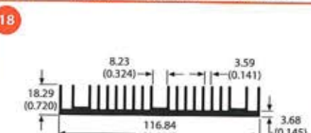
67870 1.5 lb/ft 3.37 °C/W/3in Per.=20.74
