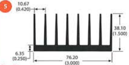
class A 64800 1.9 lb/ft 2.72 °C/W/3in Per.=25.74
