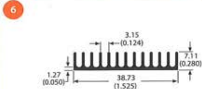
79925 0.7 lb/ft 5.98 °C/W/3in Per.=11.69
