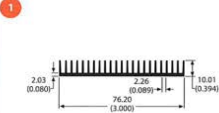
81275 0.6 lb/ft 3.49 °C/W/3in Per.=20.03
