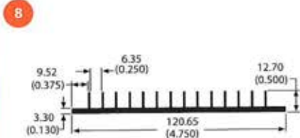
65350 1.0 lb/ft 3.50 °C/W/3in Per.=20.00
