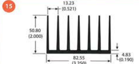
60770 2.3 lb/ft 2.23 °C/W/3in Per.=31.36
