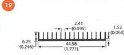
60365 1.2 lb/ft 4.51 °C/W/3in Per.=15.50
