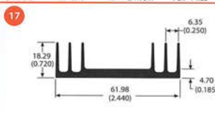
60985 0.7 lb/ft 5.99 °C/W/3in Per.=11.67
