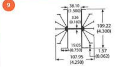
61175 2.3 lb/ft 1.25 °C/W/3in Per.=55.91
