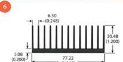
67655 1.7 lb/ft 2.21 °C/W/3in Per.=31.70
