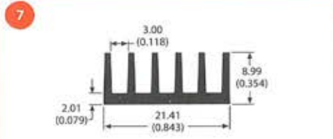
72330 0.2 lb/ft 13.94 °C/W/3in Per.=5.01
