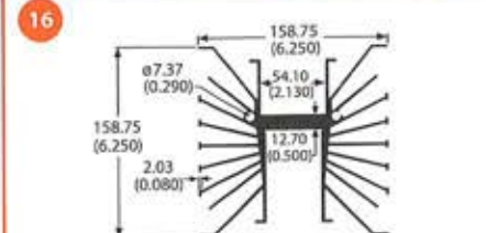
79240 7.6 lb/ft 0.65 °C/W/3in Per.=108.30
