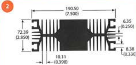
63880 14.9 lb/ft 0.78 °C/W/3in Per.=89.61
