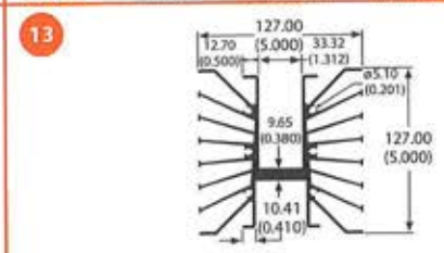
60260 5.4 lb/ft 0.84 °C/W/3in Per.=83.53
