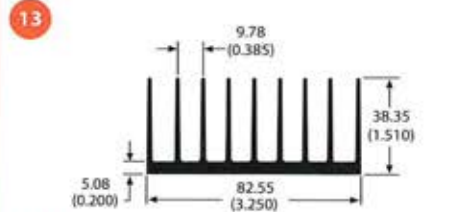
60765 1.8 lb/ft 2.35 °C/W/3in Per.=29.79
