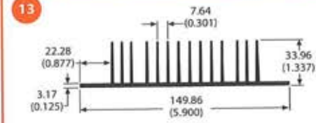
75700 2.3 lb/ft 1.56 °C/W/3in Per.=44.89
