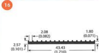
80190 0.2 lb/ft 16.96 °C/W/3in Per.=4.12
