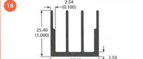
80765 0.4 lb/ft 7.61 °C/W/3in Per.=9.19
