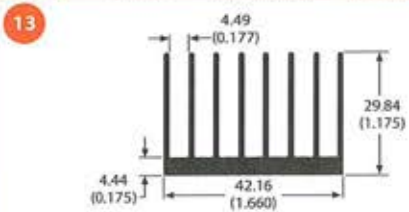
69755 0.8 lb/ft 3.60 °C/W/3in Per.=19.43
