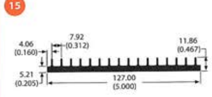
62620 1.5 lb/ft 3.89 °C/W/3in Per.=17.97
