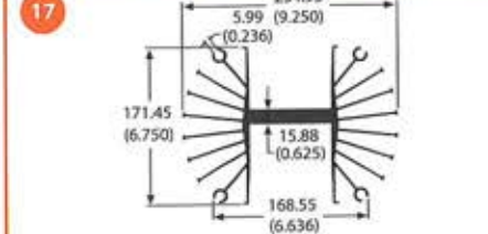
61015 9.6 lb/ft 0.60 °C/W/3in Per.=117.39
