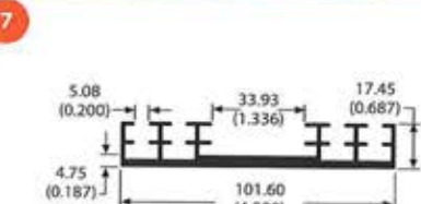
61445 1.1 lb/ft 4.13 °C/W/3in Per.=16.94
