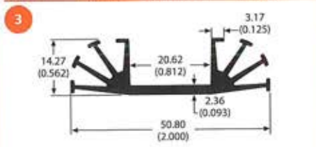
60070 0.4 lb/ft 6.96 °C/W/3in Per.=10.05
