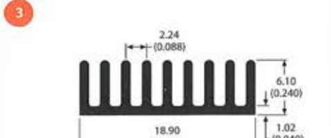
61995 0.1 lb/ft 14.24 °C/W/3in Per.=4.91
