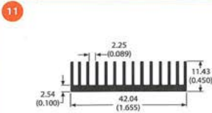
82495 0.4 lb/ft 5.35 °C/W/3in Per.=13.07
