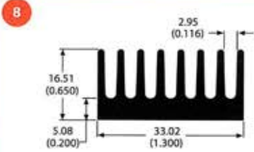
81130 0.6 lb/ft 7.31 °C/W/3in Per.=9.57
