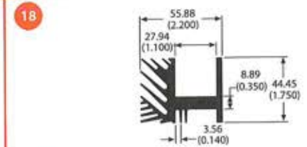
62165 1.9 lb/ft 3.4 °C/W/3in Per.=20.50
