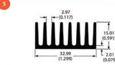
80720 0.5 lb/ft 6.81 °C/W/3in Per.=10.27
