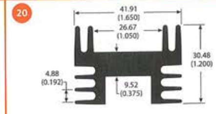
60525 1.1 lb/ft 5.85 °C/W/3in Per.=11.95
