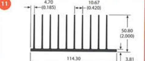
77290 2.3 lb/ft 1.54 °C/W/3in Per.=45.33
