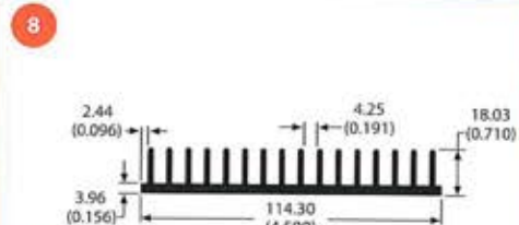
class A 65330 1.7 lb/ft 2.66 °C/W/3in Per.=26.29
