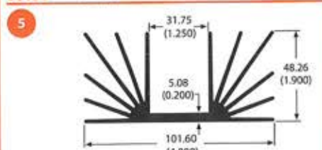
60150 1.7 lb/ft 2.46 °C/W/3in Per.=28.37
