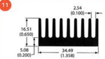
80250 0.6 lb/ft 6.61 °C/W/3in Per.=10.57
