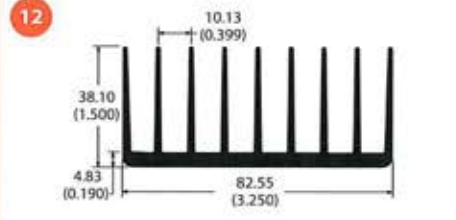
80695 1.8 lb/ft 2.35 °C/W/3in Per.=29.71
