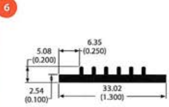
74200 0.2 lb/ft 17.95 °C/W/3in Per.=3.90
