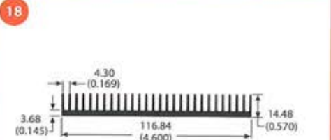
72085 1.5 lb/ft 2.20 °C/W/3in Per.=31.72
