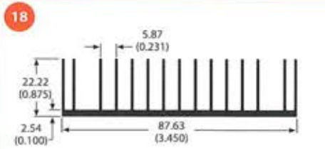
81525 0.9 lb/ft 2.31 °C/W/3in Per.=30.23
