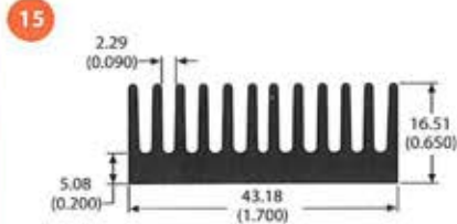
80220 0.8 lb/ft 5.07 °C/W/3in Per.=13.78
