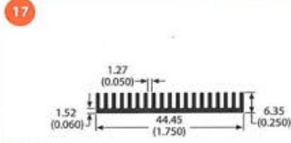
class A 65060 0.3 lb/ft 6.65 °C/W/3in Per.=10.51
