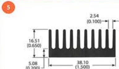
79925 0.7 lb/ft 5.98 °C/W/3in Per.=11.69
