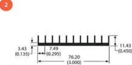
67260 0.7 lb/ft 5.33 °C/W/3in Per.=13.11
