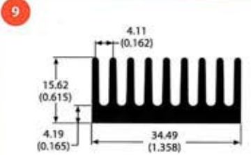
80445 0.6 lb/ft 6.61 °C/W/3in Per.=10.57
