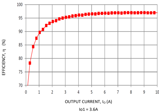
Fig 9a: Efficiency
