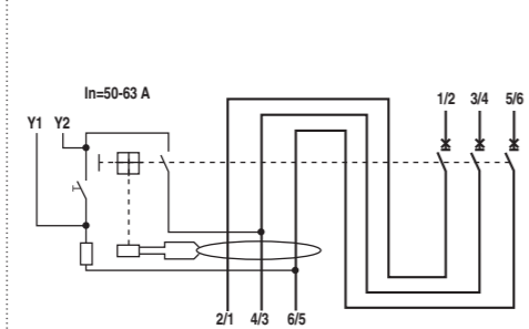
DS 203
