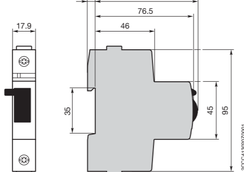
S800-NT
