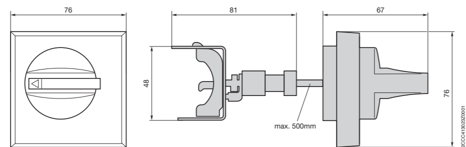
S800-RD+S800-RHE
