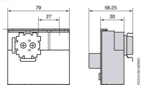
S800-BBPC120
