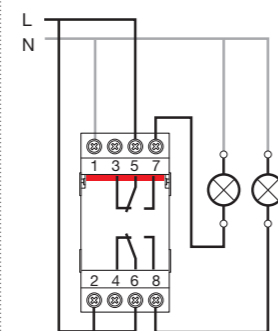
TWA-2
