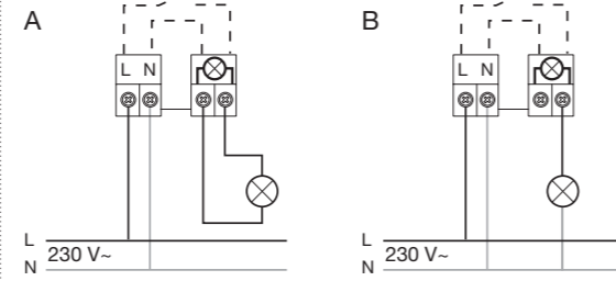
TWA-2
