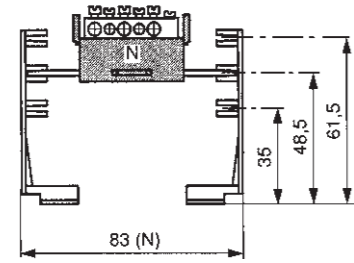
SMO 10
