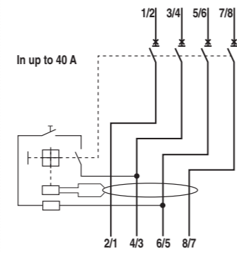
DS 204
