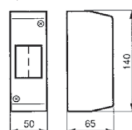
PCD 2 N
