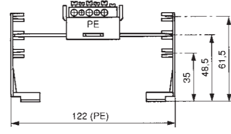
SMO 6
