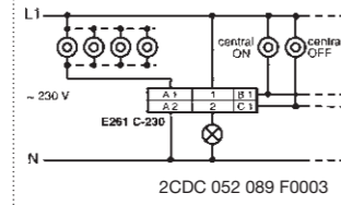
E 261 C-230
