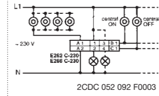
E 266 C-230
