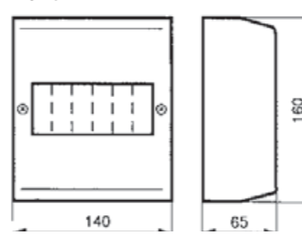
PCD 6 N
