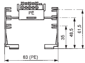
SMO 4
