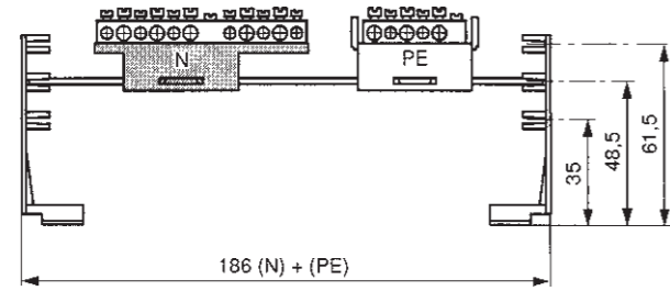
SMO 10
