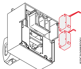
预先动作辅助触头
