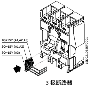
3 极断路器
