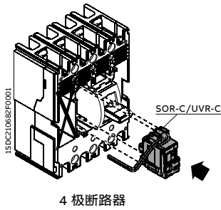
4 极断路器
