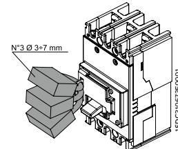
固定式分闸位置挂锁
