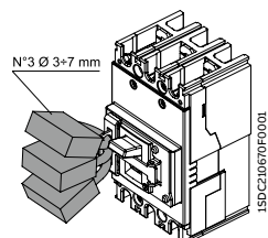
固定式分合闸位置挂锁
