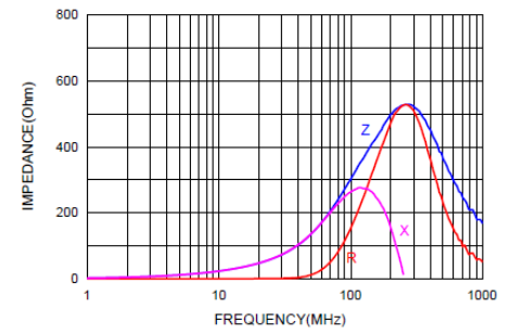
AFBC-Q0805G-301
