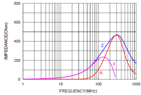
AFBC-Q0805G-221
