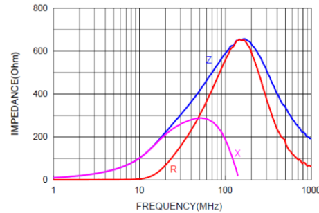
AFBC-Q0805H-601
