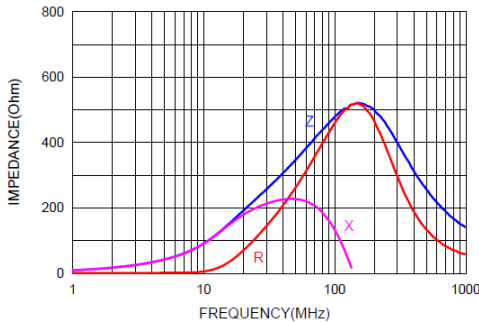
AFBC-Q0805H-471
