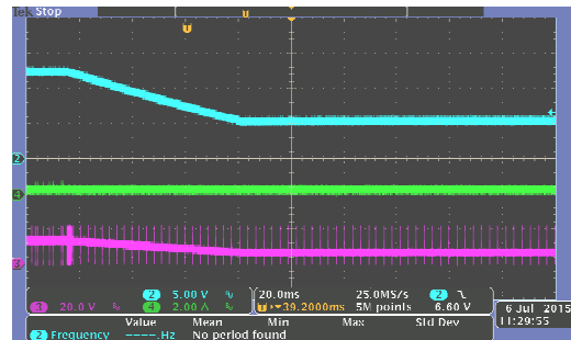
Vin=12V,Iout=0A,Vout 12V—>5V
