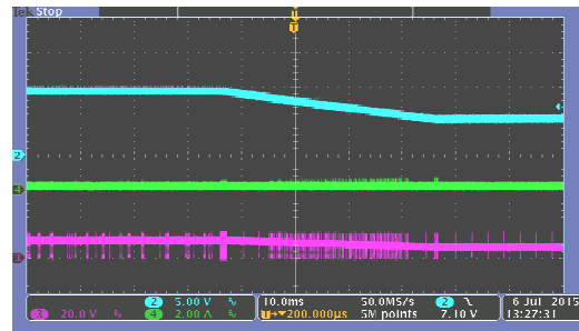
Vin=12V,Iout=0A,Vout 9V—>5V
