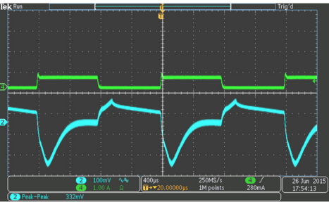
Vin=24V, load step 0A-0.5A -0A
