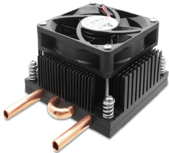
ATS-LQHS-74030-C1-R0 74.0 x 74.0 x 30.8mm Thermal Resistance: 0.13°C/W
