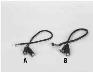
A. P/N 1703050306 Wire 30 cm 5P TV-out (S-Video, Comp. -Video)
