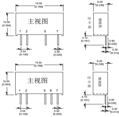
封装尺寸图
