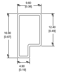
注: 单位 (Unit) : mm[inch] 未注明公差 : x.x±0.5mm[x.x±0.020inch] 0.x±0.2mm[x.x±0.008inch] 管长: 220mm[8.66inch] 包装数量: 17pcs 内盒: 235*160*82mm 包装: 9管*5层 外箱: 335*225*280mm 包装: 6盒*1箱
