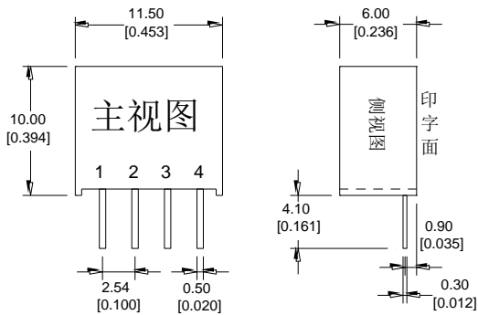
封装尺寸图
