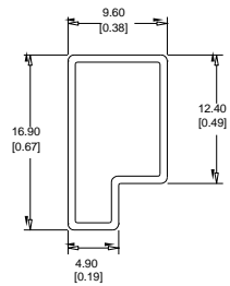
注: 单位 (Unit) : mm[inch] 未注明公差: x.x±0.5mm[x.x±0.020inch] 0.x±0.2mm[x.x±0.008inch] 管长: 220mm[8.66inch] 包装数量: 10pcs 内盒: 235*160*82mm 包装: 9管*5层 外箱: 335*225*280mm 包装: 6盒*1箱
