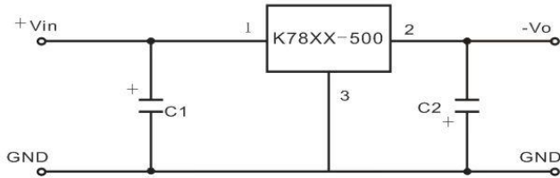
图2 负输出应用电路
