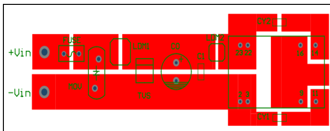
双路产品推荐电路
