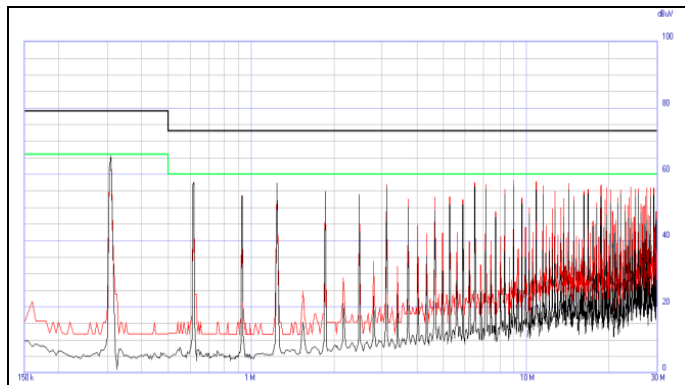
UD6-18S12E3 传导骚扰电源正极测试结果
