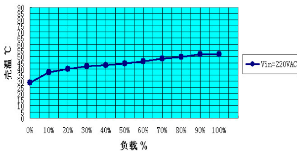
温度曲线
