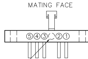
RECEPTACLE MA-1E1-005-435-A0300
