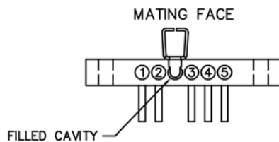
PLUG MA-1D1-005-325-A0300
