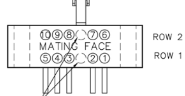
RECEPTACLE MA-281-010-435-ALC00
