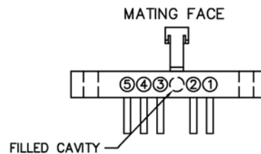
RECEPTACLE MA-1E1-005-435-A0300
