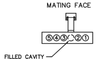
RECEPTACLE MA-141-005-261-A03WA
