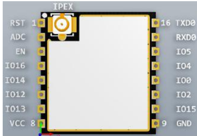
图 2 ESP-07S 管脚图
