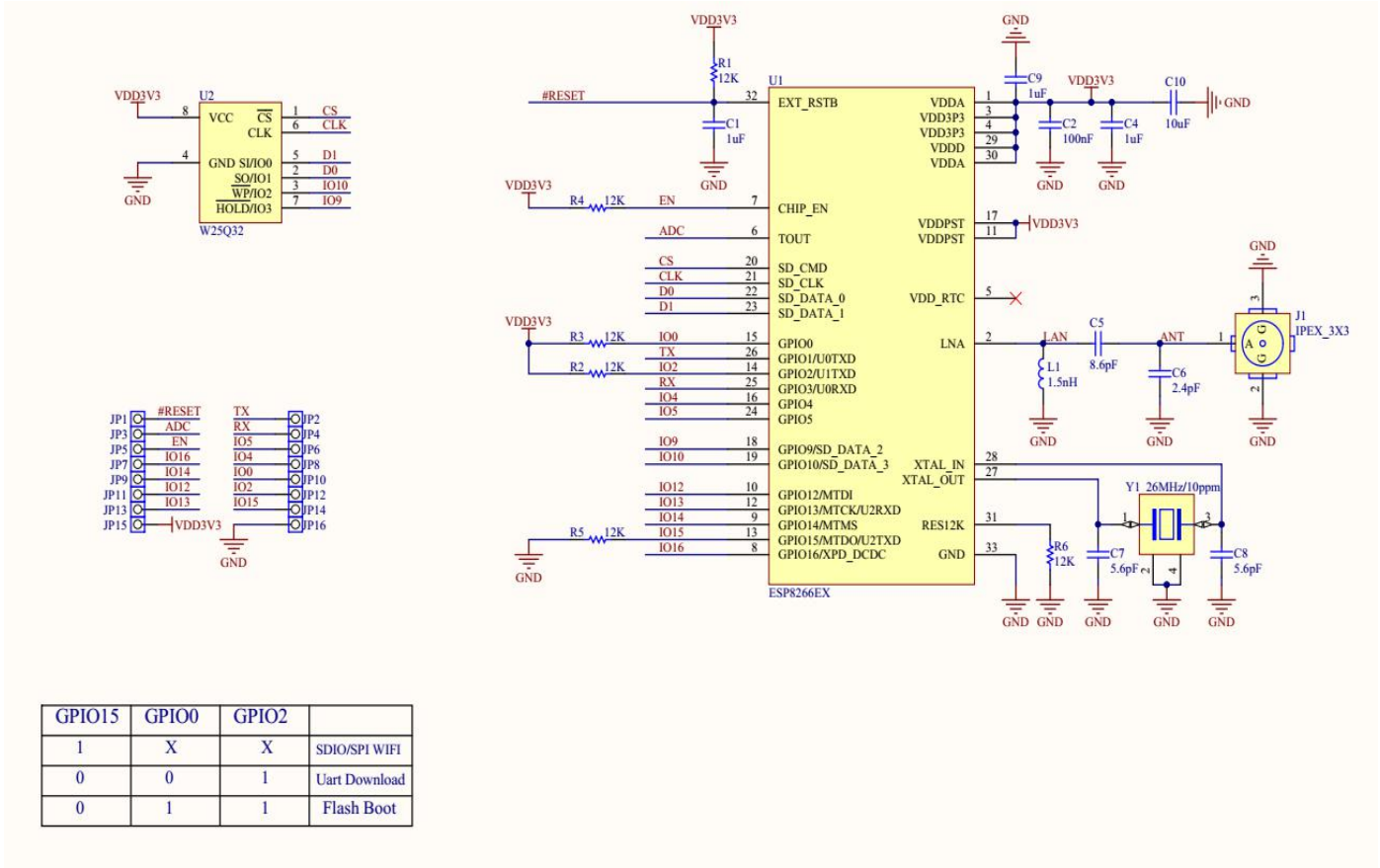
图 5 ESP-07S 原理图
