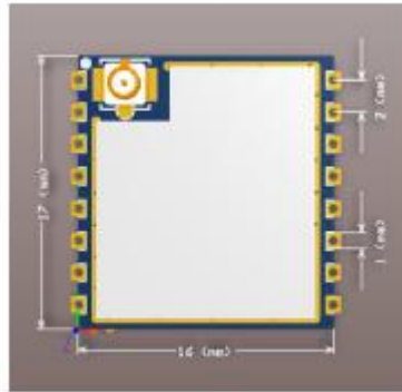
ESP-07S 模组尺寸平面面图
