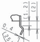
取付板のスナップ部詳細 RETENTION FEATURE DETAIL
