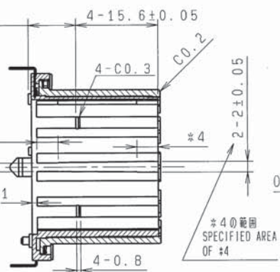
断面YY SECTION YY
