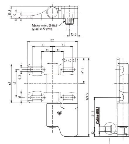
SHS3...KR...
