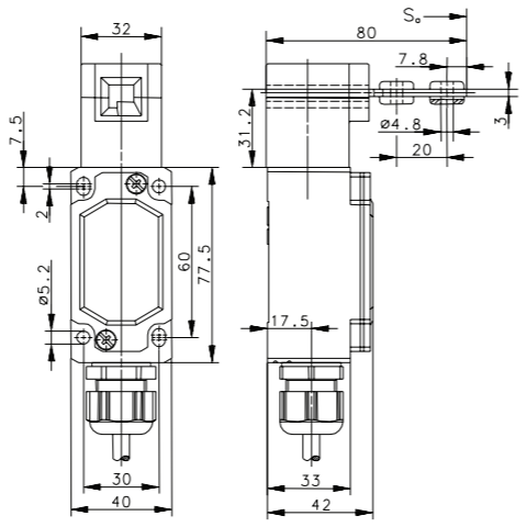
ENM2 VTW
