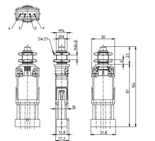
IWF AMP4
