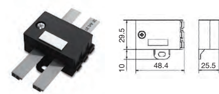
607.3900.047 ASI CABLE LINK
