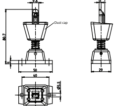
A3 ACTUATOR KEY 391.1702.230
