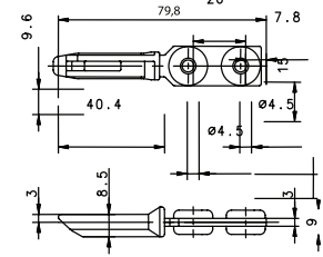
A1 ACTUATOR KEY 391.1702.228
